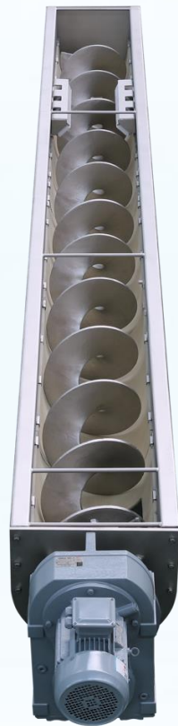
无轴螺旋输送机
