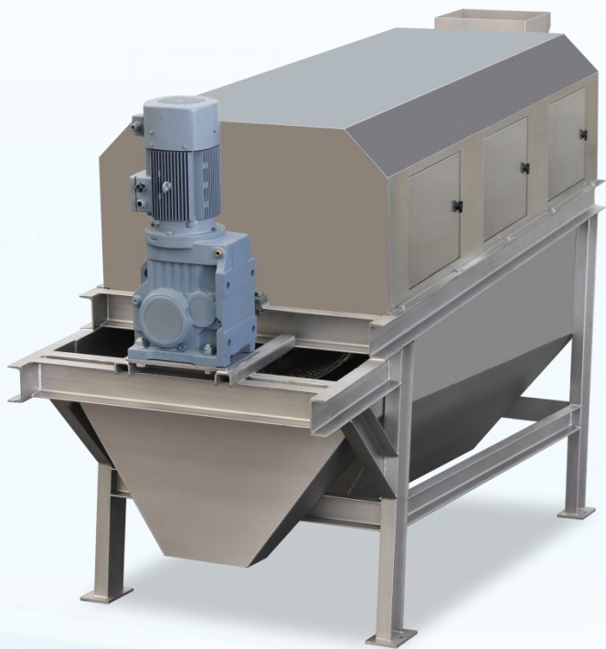
景津滤饼除杂机
